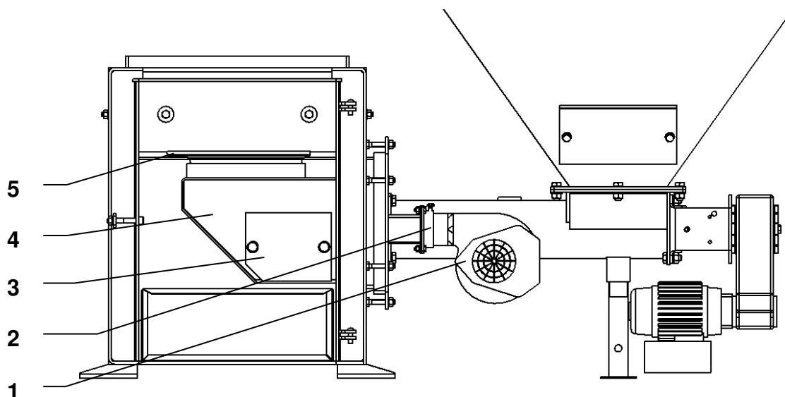
Obr. č. 4 Spalovací komora setu
